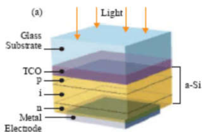
圖 1.2-5、Superstrate 結構
