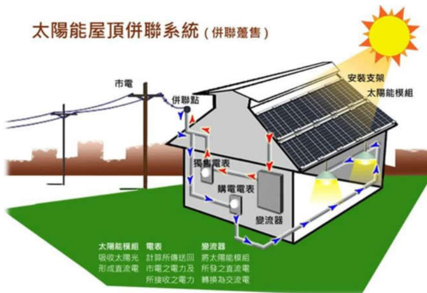
圖 1.1-12、太陽光電系統與市電並聯示意圖 21
