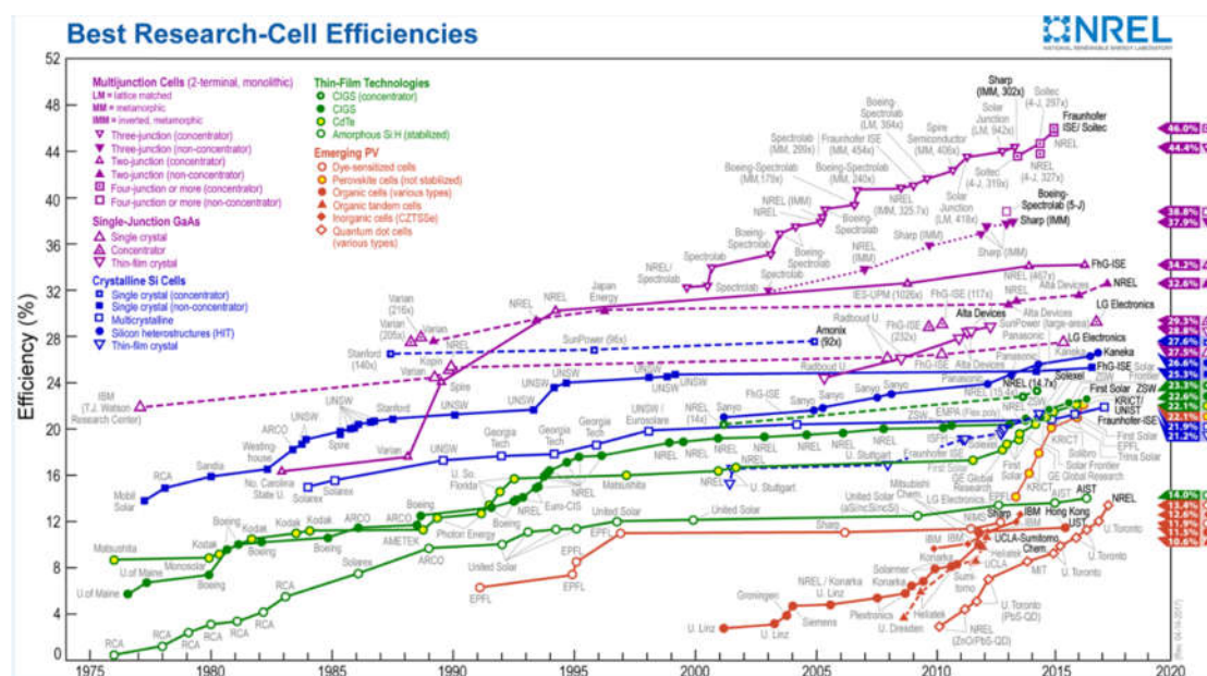
圖 1.1-10、各類太陽能電池之光電轉換效率 19
