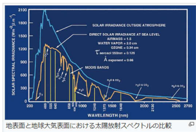
圖 1.1-3、太陽光譜圖 11
