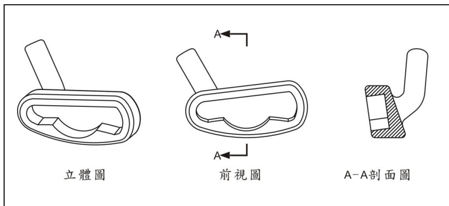
圖 1-11 高爾夫球桿之桿頭
