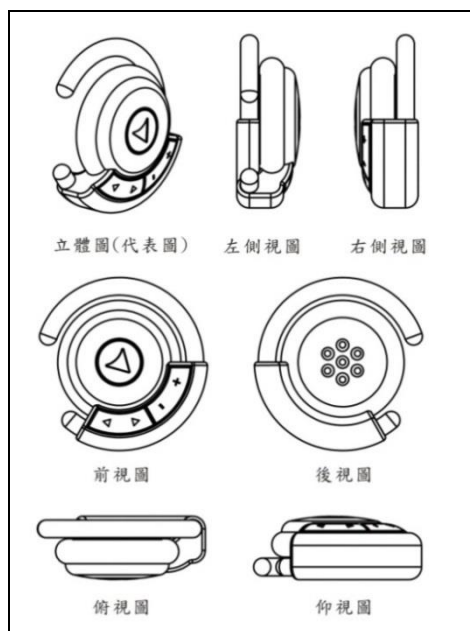
圖 1-6 立體圖及六面視圖
