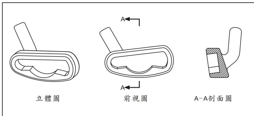
圖 1-11 高爾夫球桿之桿頭
