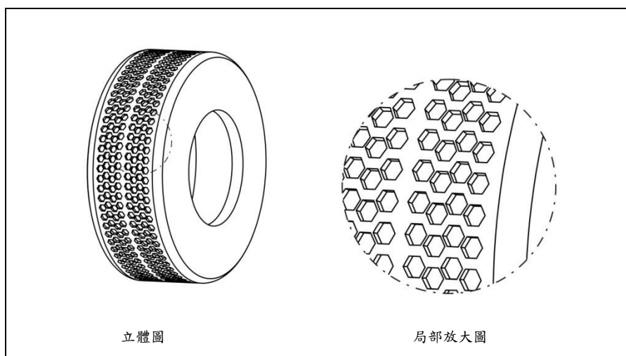
圖 1-12 輪胎
