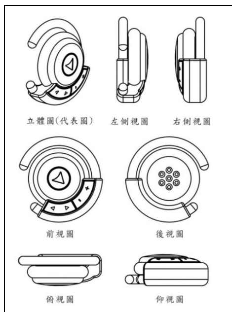
圖 1-56 立體圖及六面視圖
