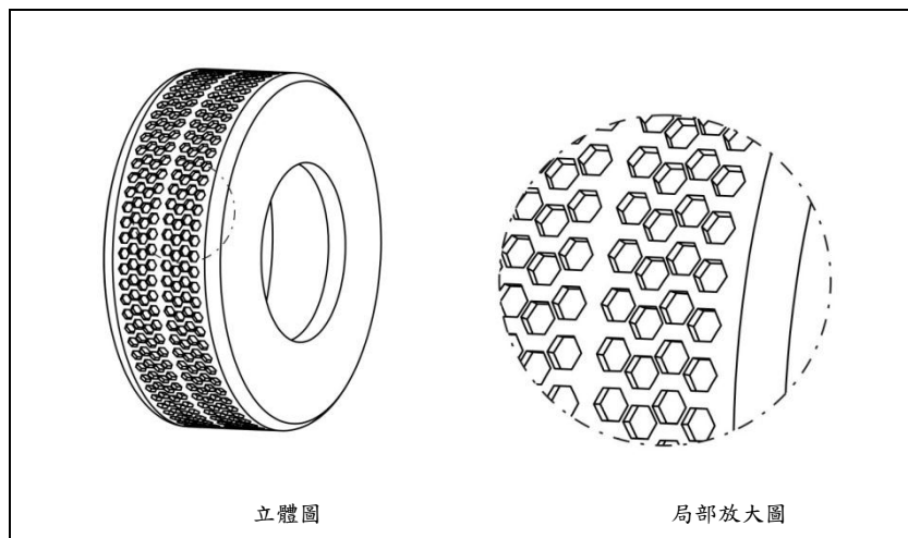
圖 1-11 輪胎
