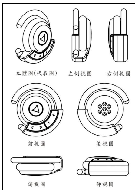
圖 1-5 立體圖及六面視圖
