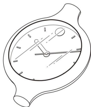
圖 1-21 具透明材質之物品的表示方式
