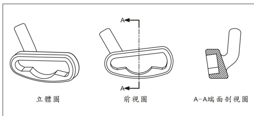
圖 1-10 高爾夫球桿之桿頭
