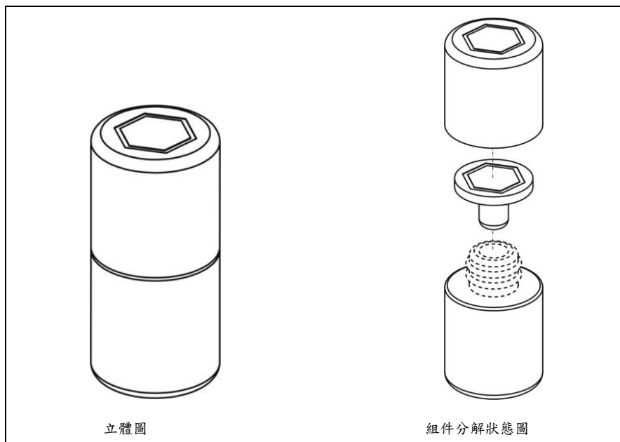
圖 7-2 容器之部分
